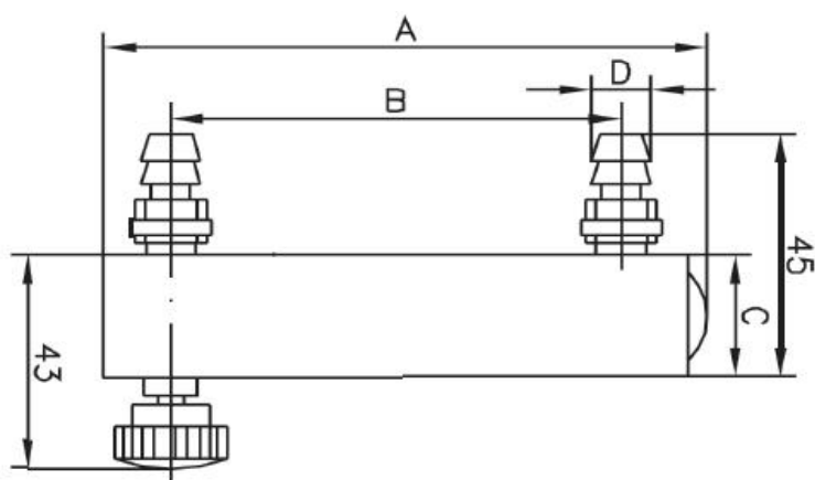
图一. LZB-4M、6M型氧吧流量计外形图
