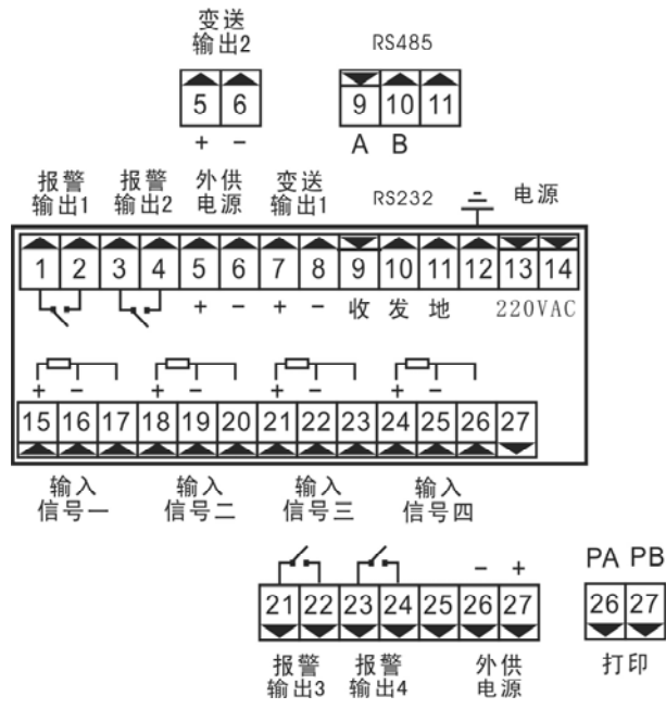
图 4.3 仪表接线端子图
