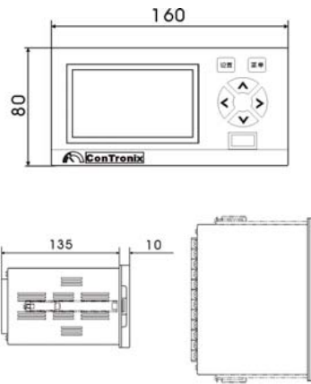
图 4.1 仪表外形尺寸
