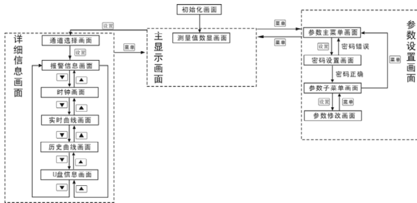
图 5.3 运行和操作流程图
