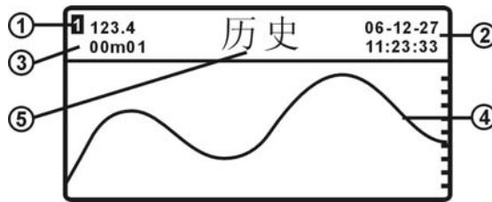
图 5.15 历史曲线画面
