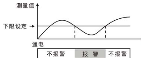
图 7.1 待机下限报警示意图
