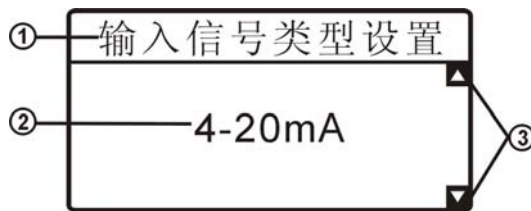
图 5.27 参数设置画面
